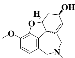
Fig. 3. Galantamine
