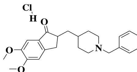
Fig. 1. Donepezil hydrochloride
