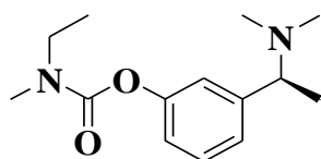
Fig. 2. Rivastigmine
